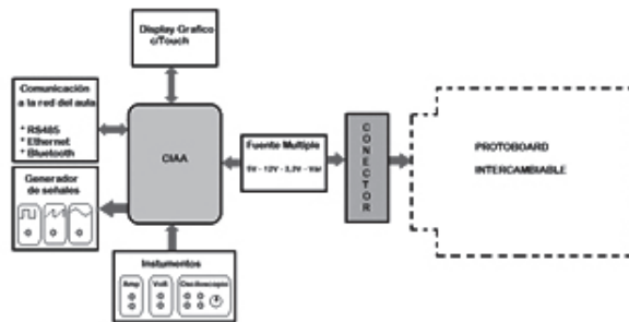
Figura 2 - Diagrama en bloques del desarrollo propuesto. (Fuente propia)
