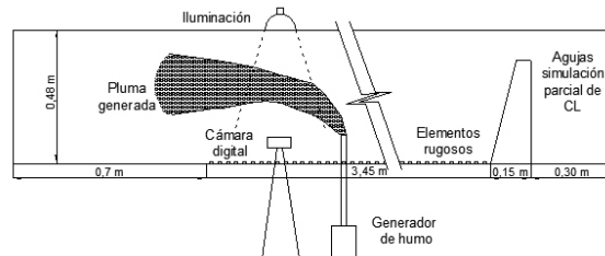
Figura 1. Disposición del instrumental durante el ensayo.
