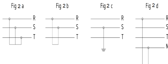
Fig. 2: Tipos de corto circuito.
